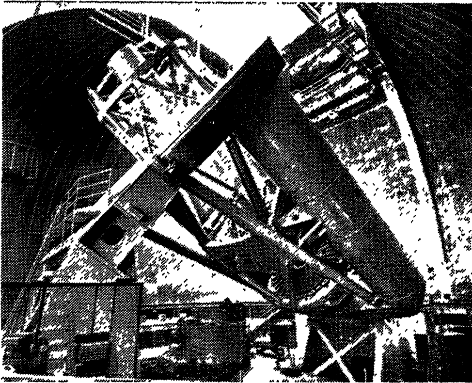
رصدخانه پالومر وابسته بدانسگاه کالیفرنیا
